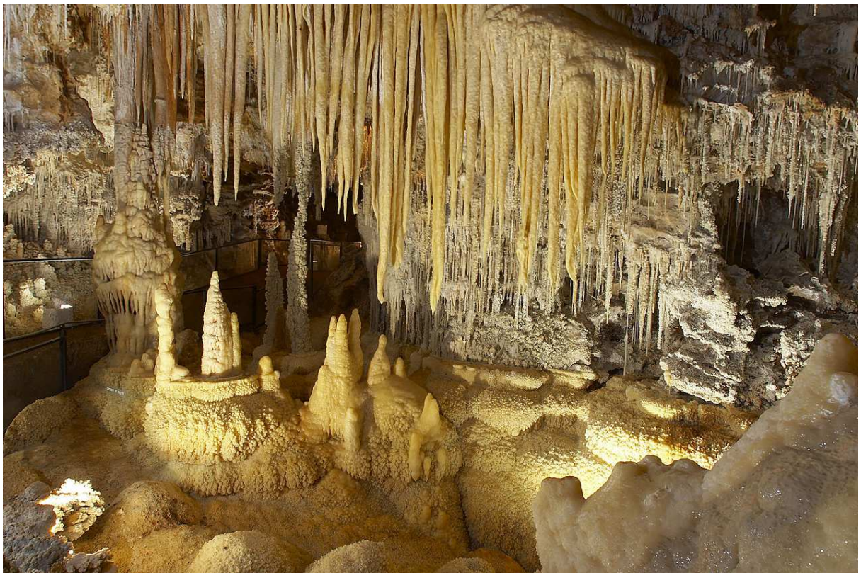
Stalactites et stalagmites dans la grotte de Niaux
